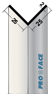
Proface®-CORNEQ CQ250-A
