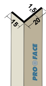
Proface®-CORNEQ CQ150N-P
