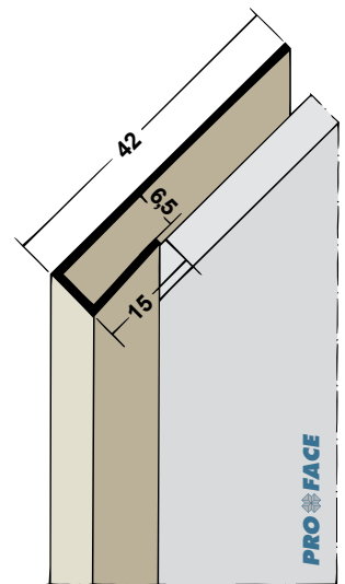
Proface®-YOIN-U U65-P
