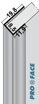
Proface®-YOIN-U U85-A
