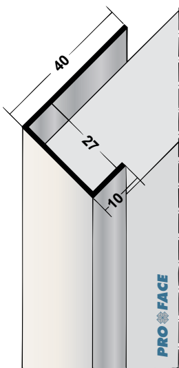
Proface®-YOIN-U U270-A
