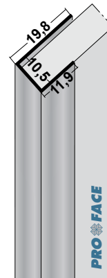
Proface®-YOIN-U U105-A
