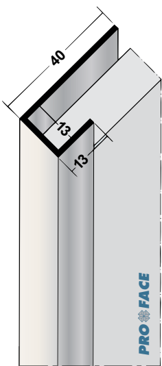
Proface®-YOIN-U U130-A
