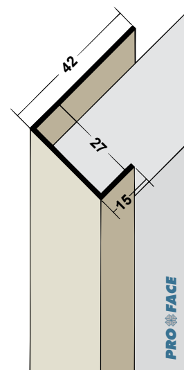
Proface®-YOIN-U U270-P
