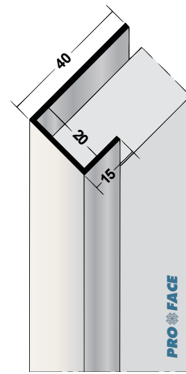
Proface®-YOIN-U U200-A
